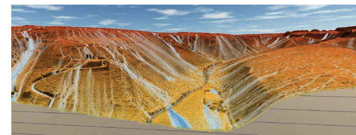
Modélisation des ruissellements dans la forêt, lors des pluies intenses : un relevé topographique par LIDAR, effectué par le SIARE en 2019, a servi de base pour identifier les axes de ruissellement au sein de la forêt afin de mener des actions de rééquilibrage des arrivées d'eau (hydraulique douce).
